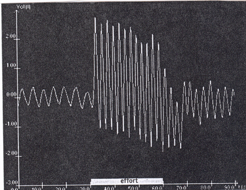
c. Enregistrement de la spirométrie chez un sujet au repos et durant un effort.
